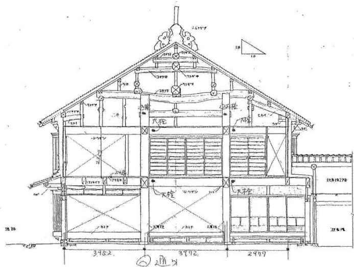
重要文化財 上芳我家住宅（愛媛県内子町）明治 27 年(1894) 断面
